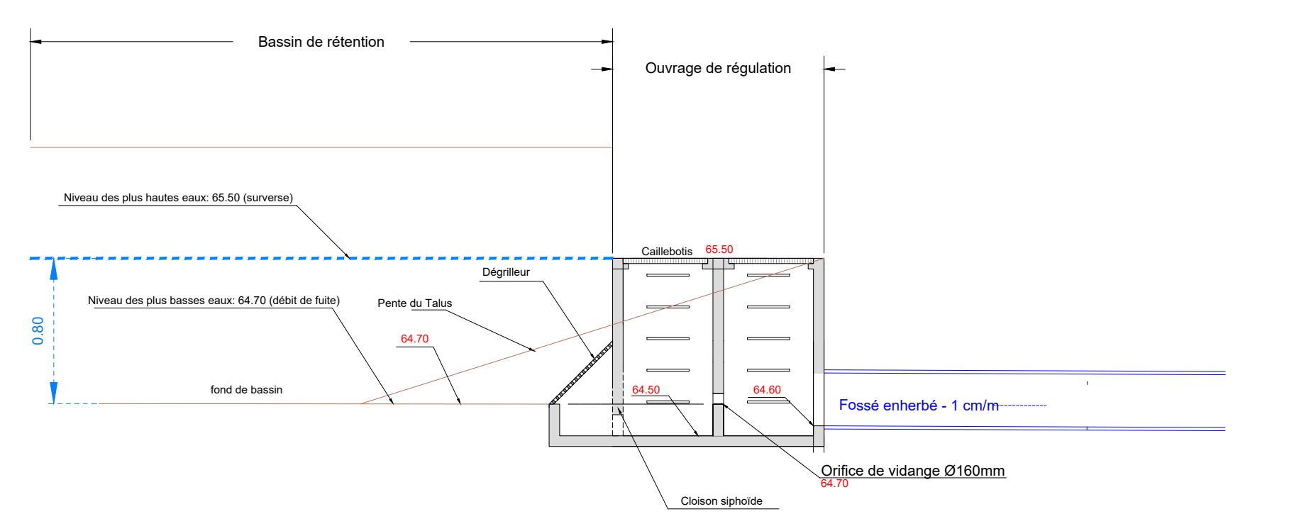
BASSIN N°2 - COUPE PRINCIPLE - OUVRAGE DE REGULATION / SURVERSE (echelle 1/50)
