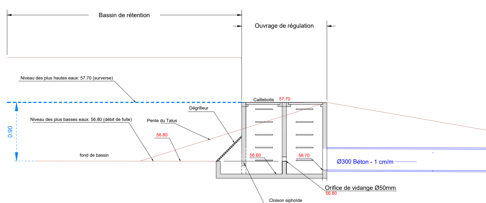
BASSIN N°5 - COUPE PRINCIPALE - OUVRAGE DE REGULATION / SURVERSE (echelle 1/50)
